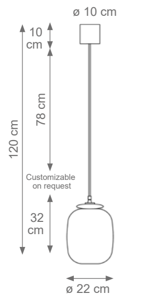
Soho Pendant Light Code: F808031 Type 1 light electrification x Max 28W E14 CE Size: cm. 32 h x 22 ø - 2,5 kg
