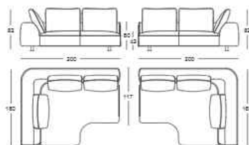
Dormeuse senza bracciolo / chaise longue without armrests / Угловой диванчик без подлокотников
