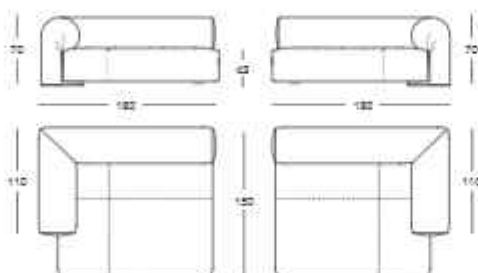
Dermaux con bracciolo / chaise longue with armrests / Угловой с подлокотниками
